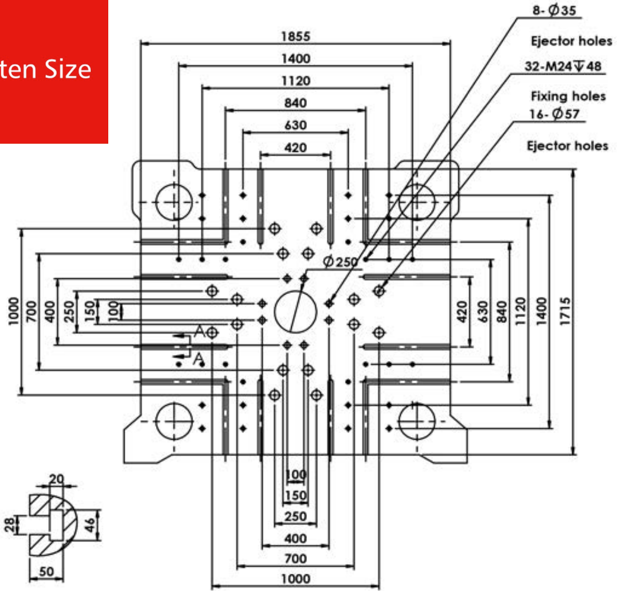
A-A T-slot
