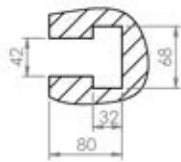
A-A T - slot
